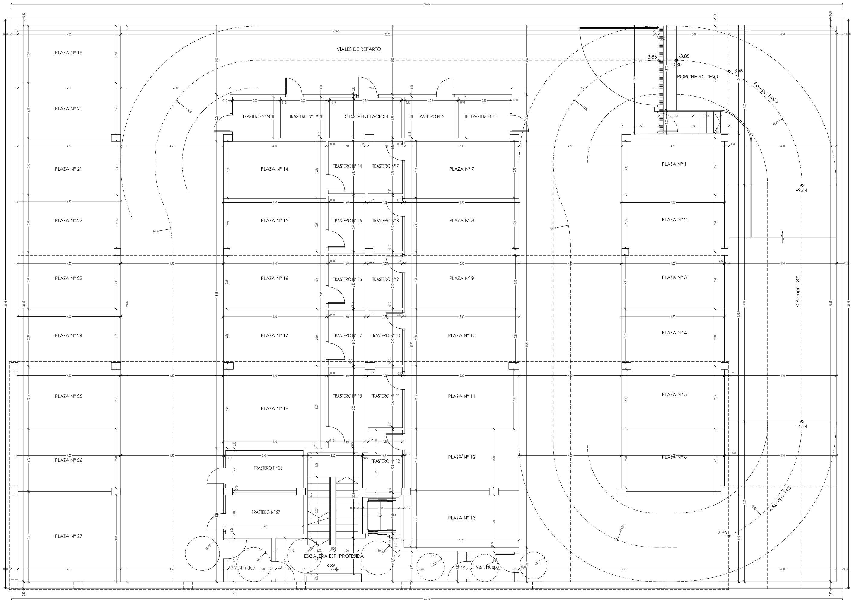
Planta sotano -1º
